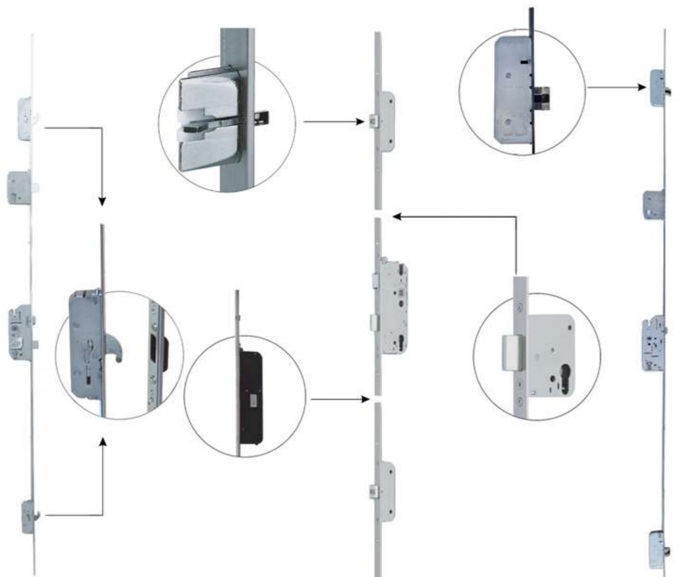
Zasuwnica FUHR haki
